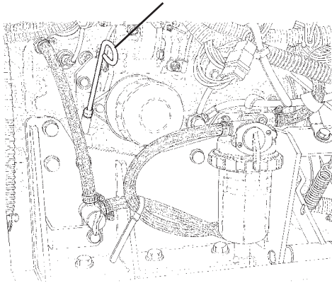
オイルレベルゲージ
