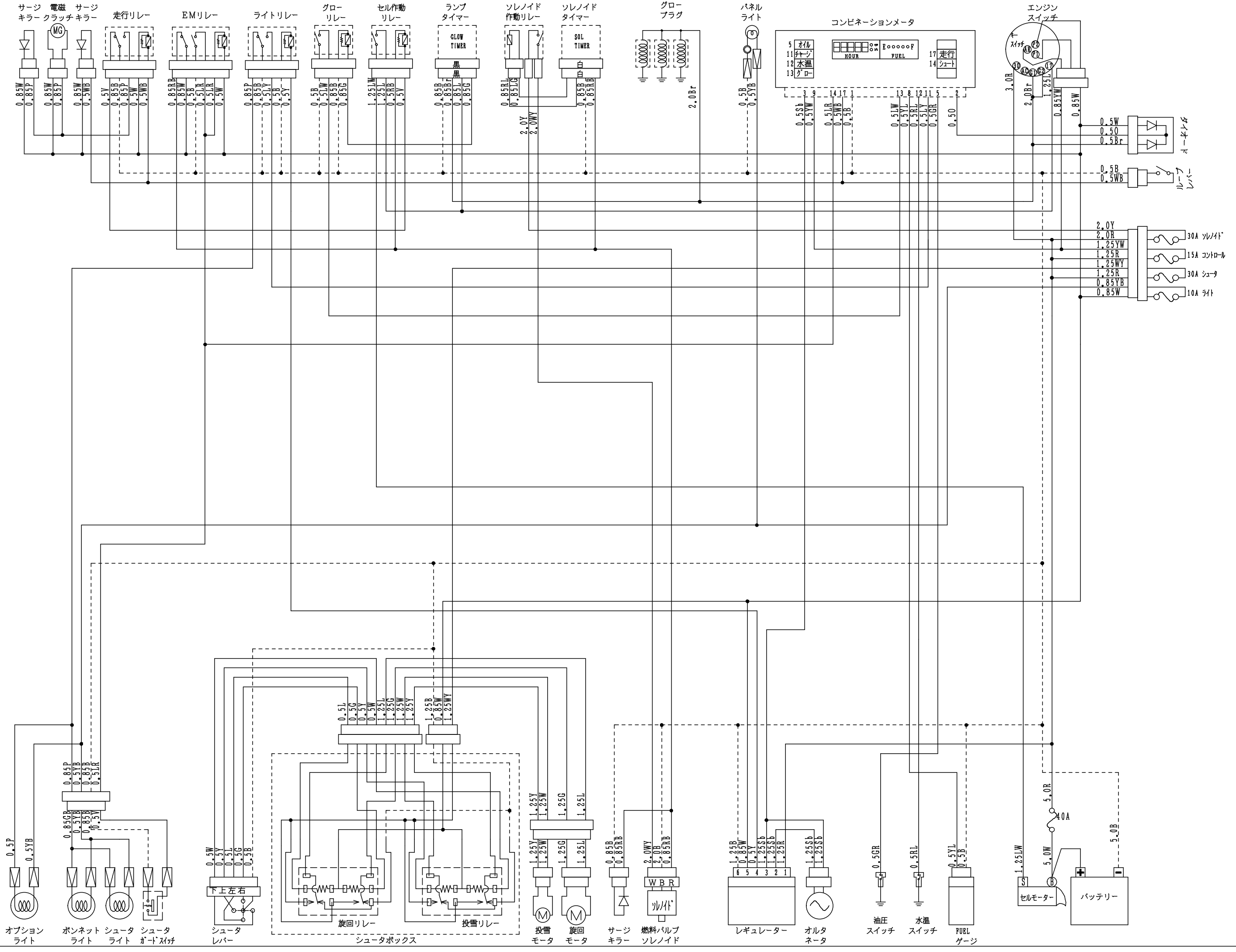
SX1510回路図
