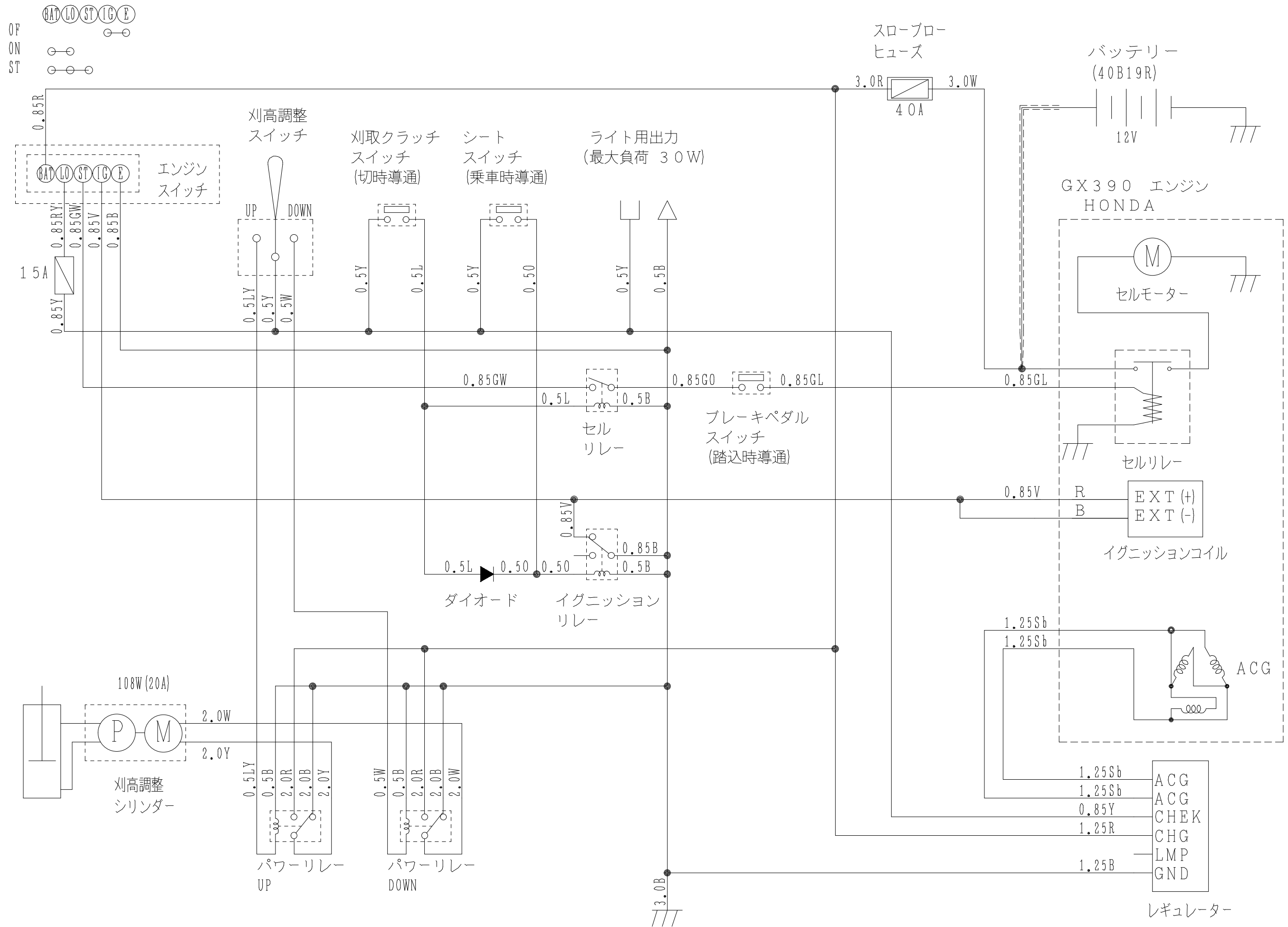
WK-2 1回路図 ('13,12,10)
