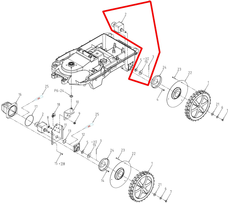
08013-M92-000 走行モーター交換KIT
