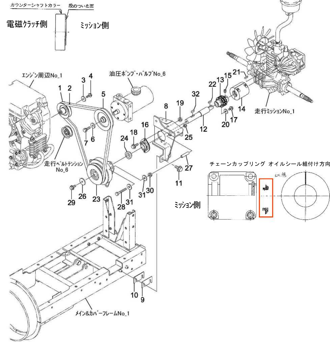
電磁クラッチ カウンターシャフトカラー (No24) 組付方向
