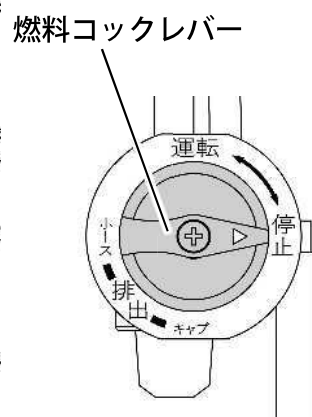
<燃料コック>
