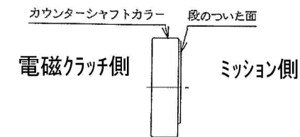
電磁クラッチ カウンターシャフトカラー (No24) 組付方向
