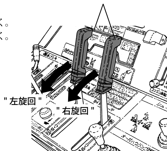
サイドクラッチレバー
