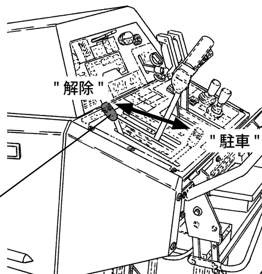
駐車ブレーキレバー
