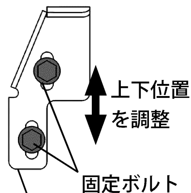
フロントブラケット 正面図（左側）
