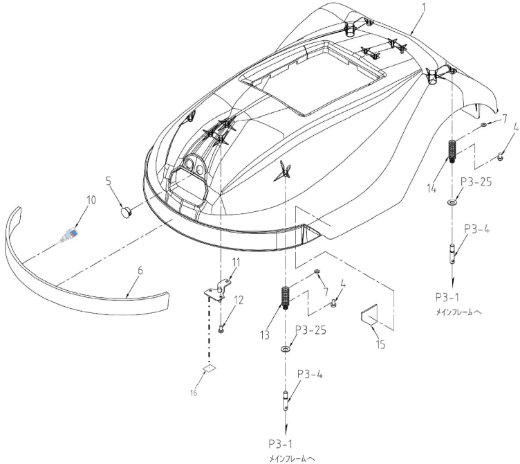
No. 1 08017-M92-030 メインカバー交換ASSY 構成
