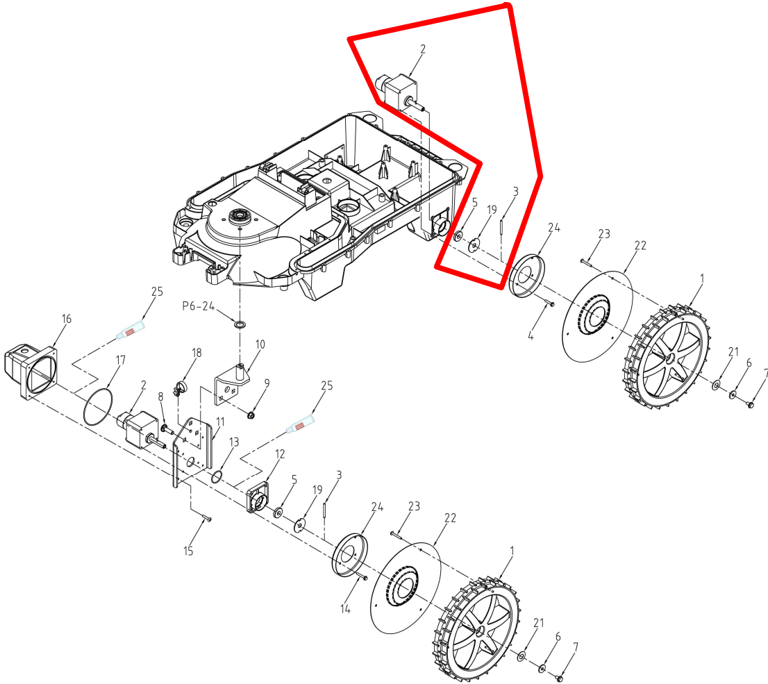
08013-M92-000 走行モーター交換KIT
